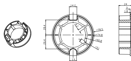
1.0405.0108 Bague d'entraînement (Moteur AM45)
