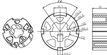
1.0405.0001 Bague d'entraînement (Moteur AM45)
