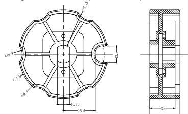
1.0405.0041 Bague d'entraînement (Moteur AM45)
