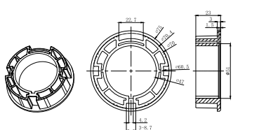
1.0405.0100 Bague de fin de course(Moteur AM45)
