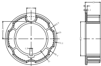
1.0405.0041 Bague d'entraînement (Moteur AM45)
