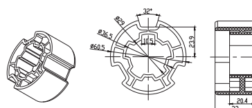
1.0405.0033 Bague d'entraînement (Moteur AM45)
