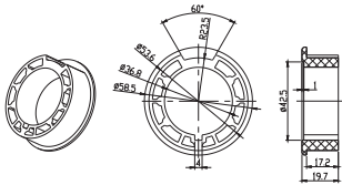
1.0404.0018 Bague de fin de course (Moteur AM35)
