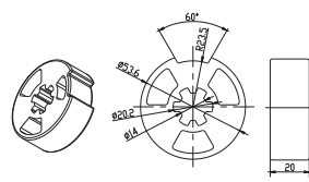
1.0404.0050 Bague d'entraînement (Moteur AM35)
