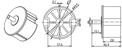
1.0404.0071 Bouchon (Moteur AM35)
