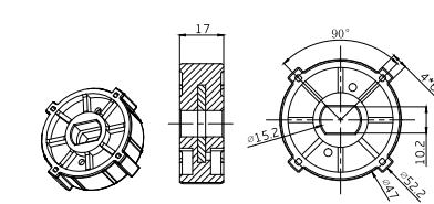
1.0404.0153 Bague d'entraînement (Moteur AM35)
