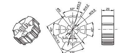
1.0404.0051 Bague d'entraînement (Moteur AM35)
