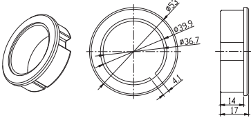
1.0404.0015 Bague de fin de course (Moteur AM35)
