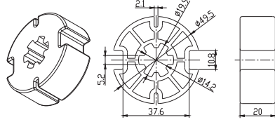
1.0404.0048 Bague d'entraînement (Moteur AM35)
