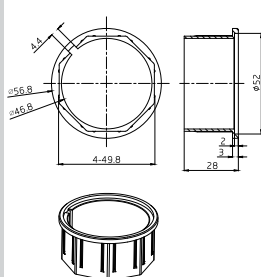
1.0405.0136 Bague de fin de course (Moteur AM45)
