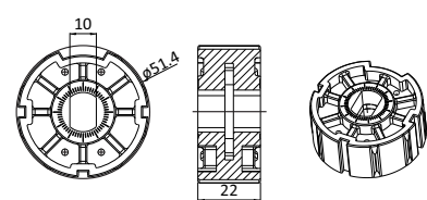
1.0404.0093 Bague d'entraînement (Moteur AM35)
